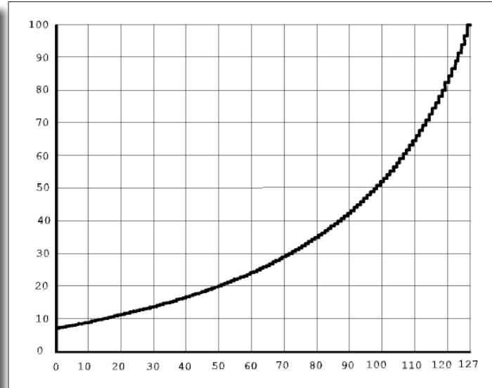
Kennlinie für die Höchstgeschwindigkeit (siehe CV05/CV61)
