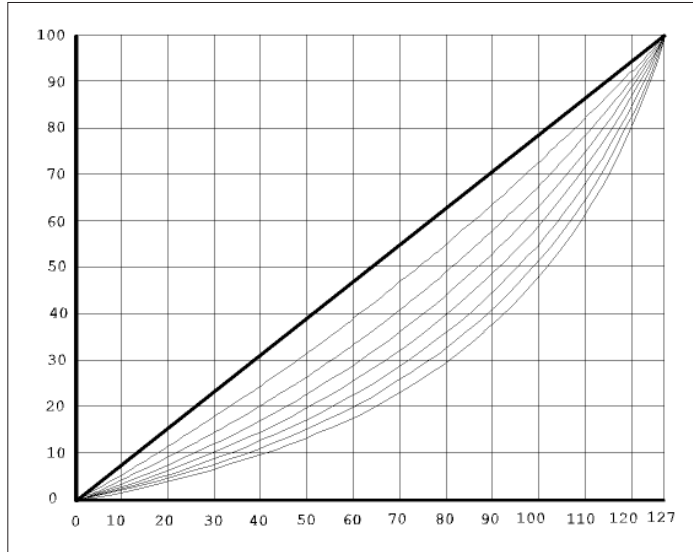
Fahrstufenkennlinie *), (siehe CV48)
